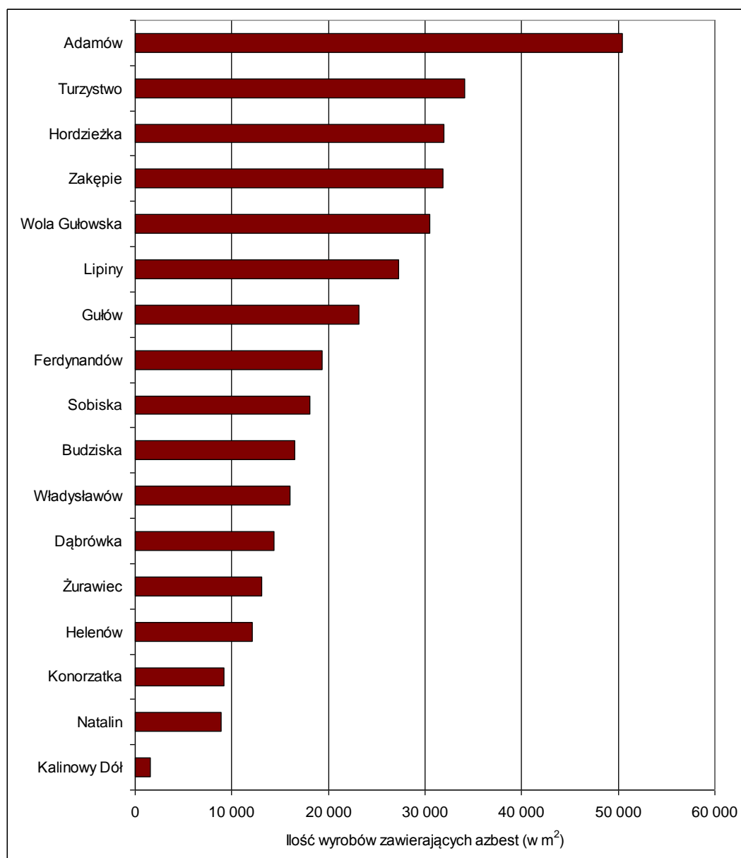
Rycina nr 3 Rozmieszczenie odpadów zawierających azbest na terenie gminy Adamów
